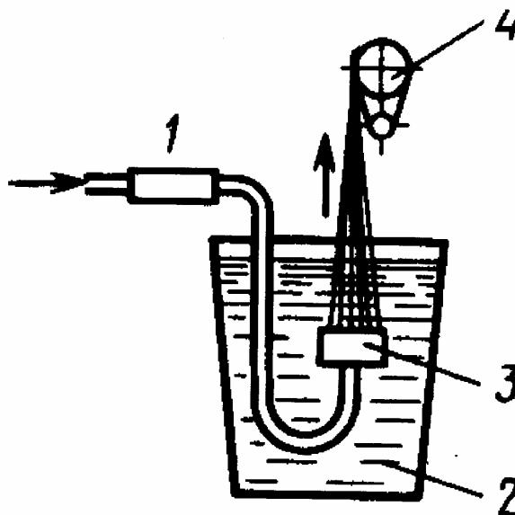
Рис. 13. Схема мокрого формования вязкого волокна
