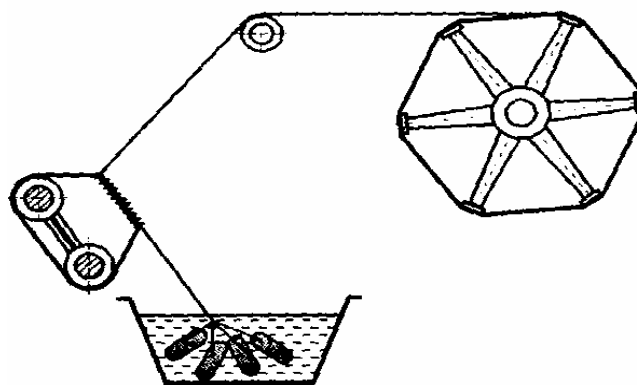
Рис. 12. Схема разматывания коконов
