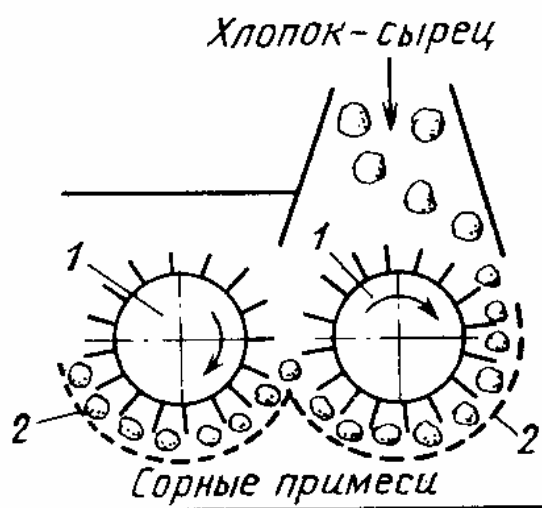
Рис.4. Схема предварительной очистки хлопка-сырца на колковых барабанах
