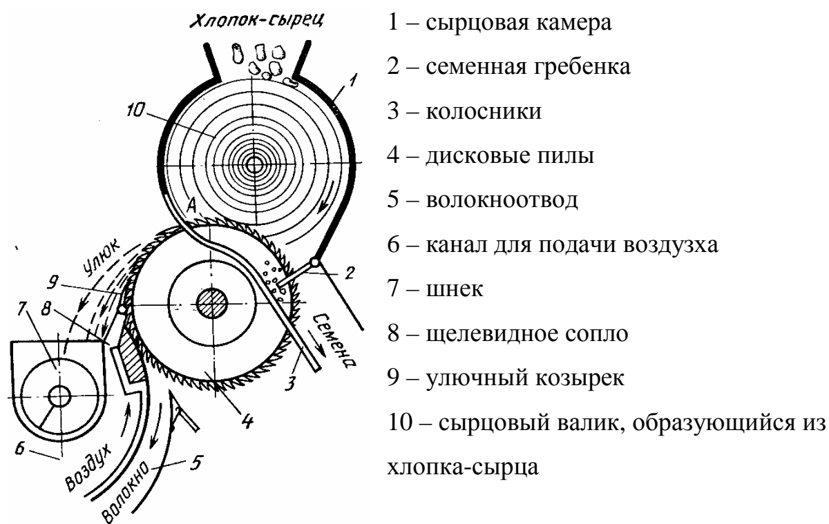
Рис. 5. Схема пильного волокноотделителя
